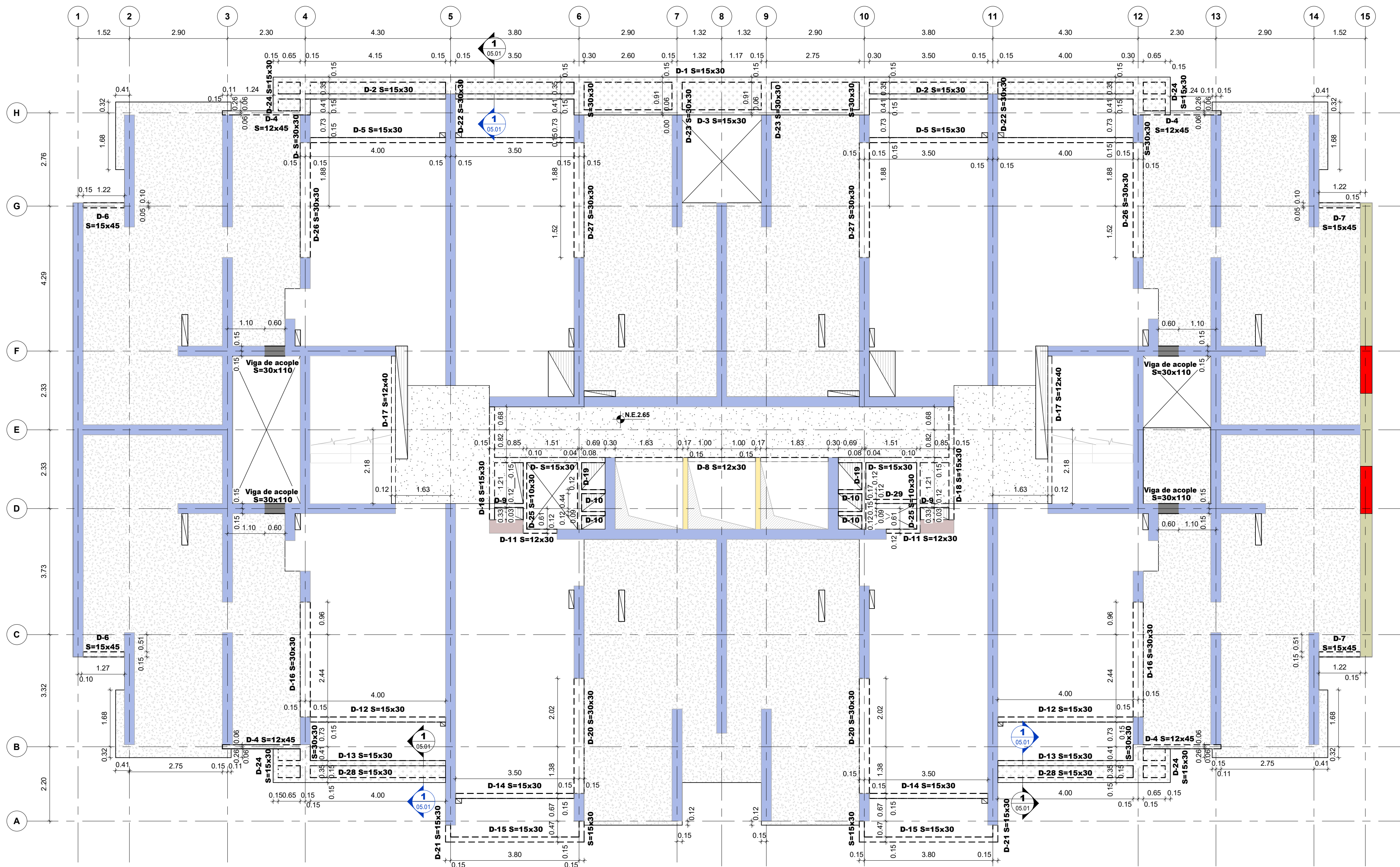
PLANTA LOCALIZACIÓN DE DINTELES PISO 2 Escala 1 : 75
