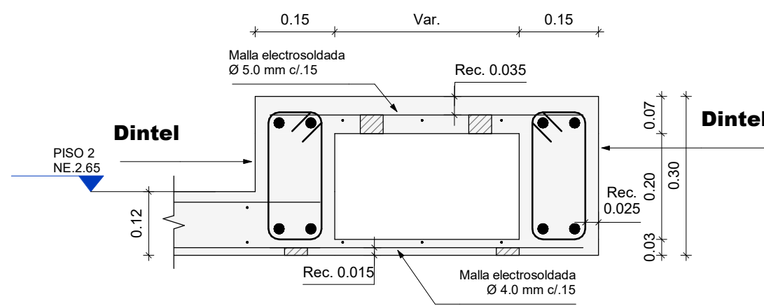
CORTE 1 - 1 PLACA ALIGERADA Escala 1 : 10
